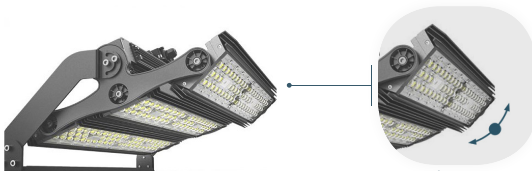
Beleuchtungsmodule einzeln schwenkbar
